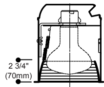
312 Baffle
