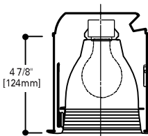
30 Baffle
